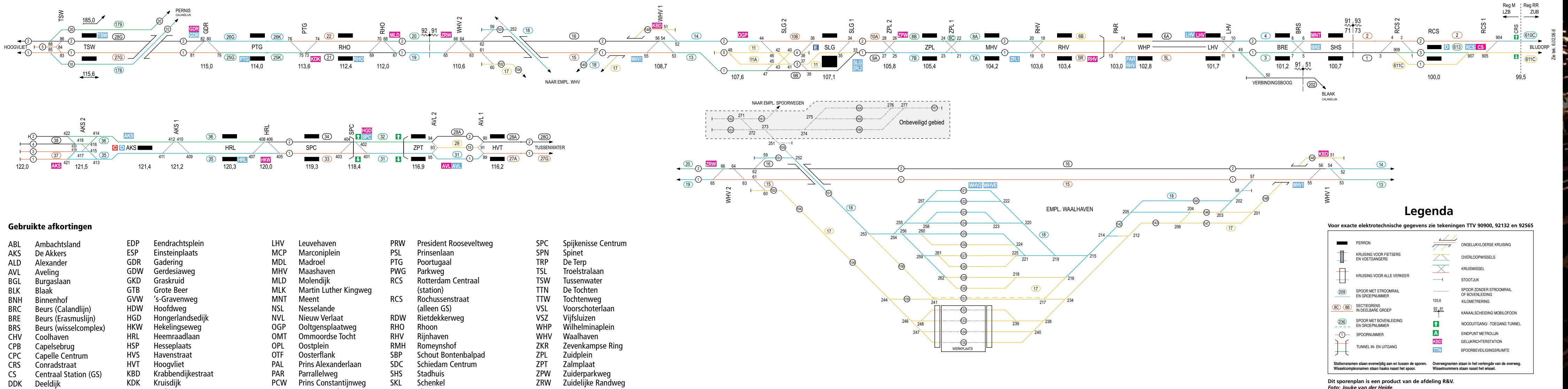
Schematisch overzicht van stations en overwegen sporen, seinen en wissels stroomrail- en bovenleidingsgroepen
